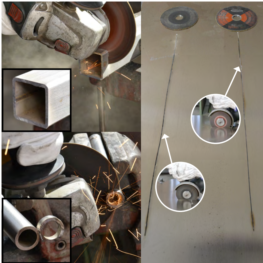
Burr-free, cool and precise cuts with GLOBE HP ONE Tagli senza bave, freddi e precisi effettuati con GLOBEHP ONE
